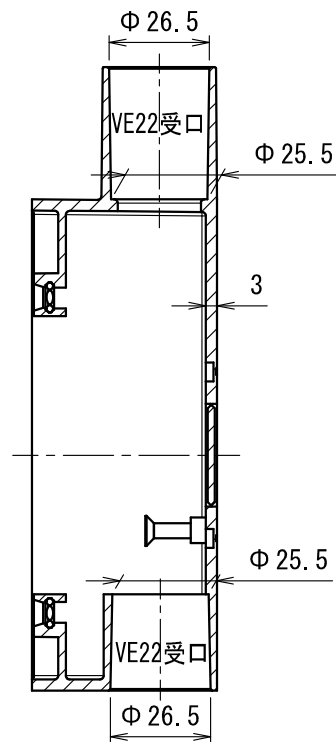
断面 A-A
